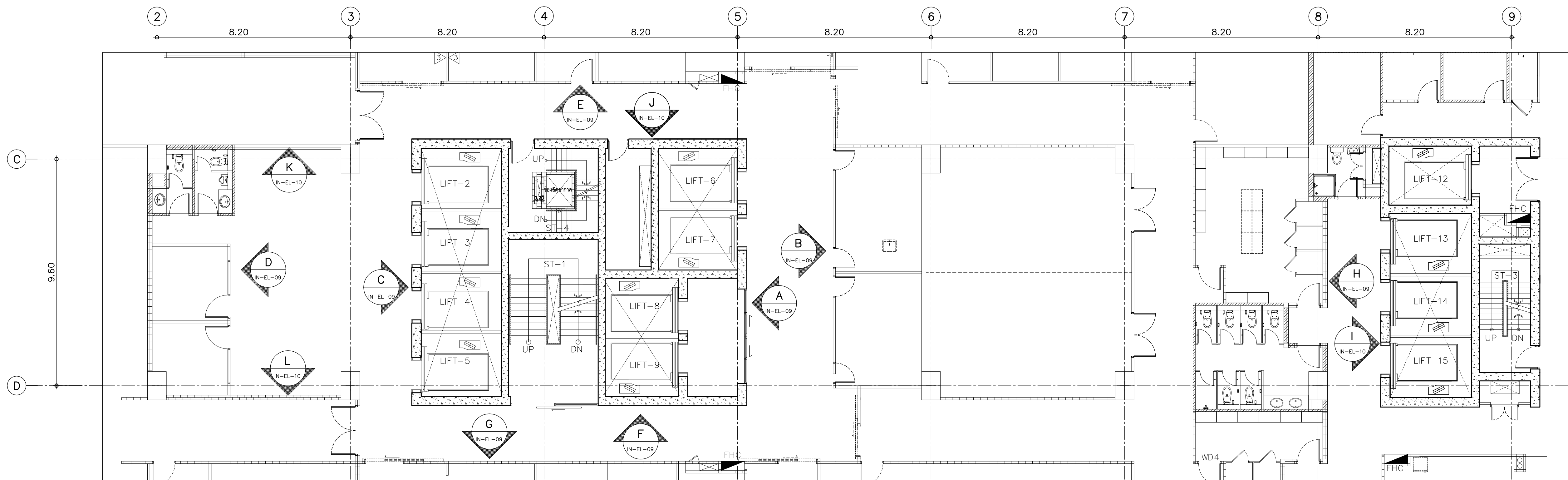
แผนผังเฟอร์นิเจอร์ชั้นที่ 6 มาตราส่วน 1:100
