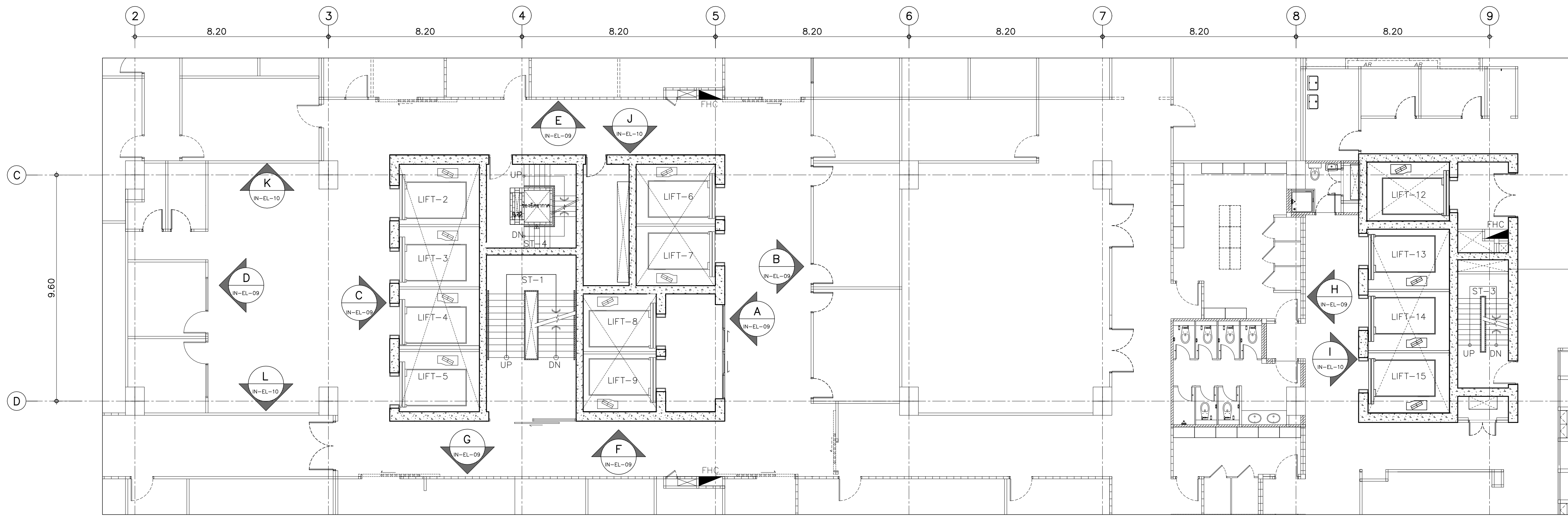
แผนผังเฟอร์นิเจอร์ชั้นที่ 7 มาตราส่วน 1:100
