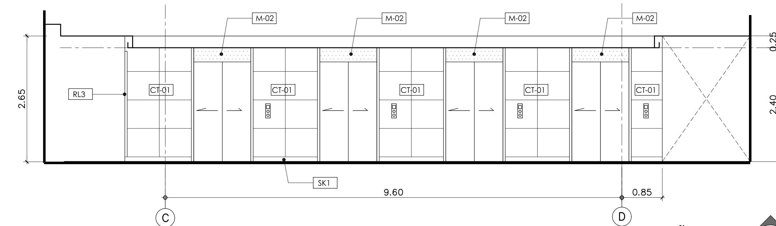
รูปด้าน มาตราส่วน 1:50 C (N-EL-11)
