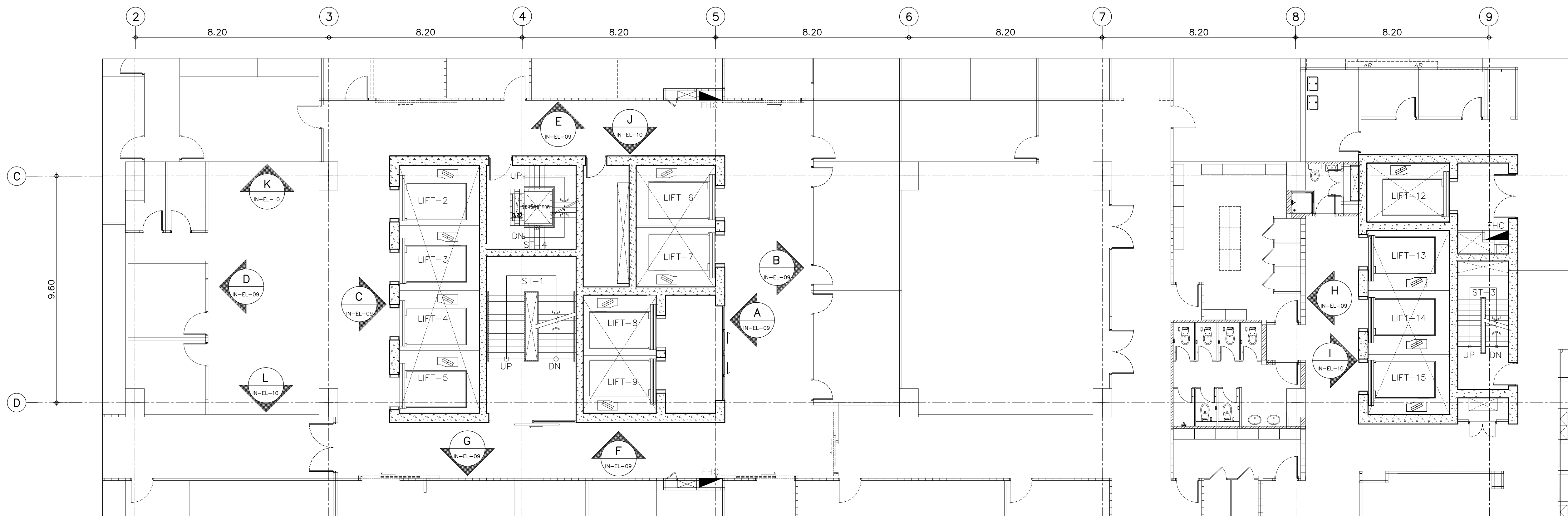
แผนผังเฟอร์นิเจอร์ชั้นที่ 5 มาตราส่วน 1:100
