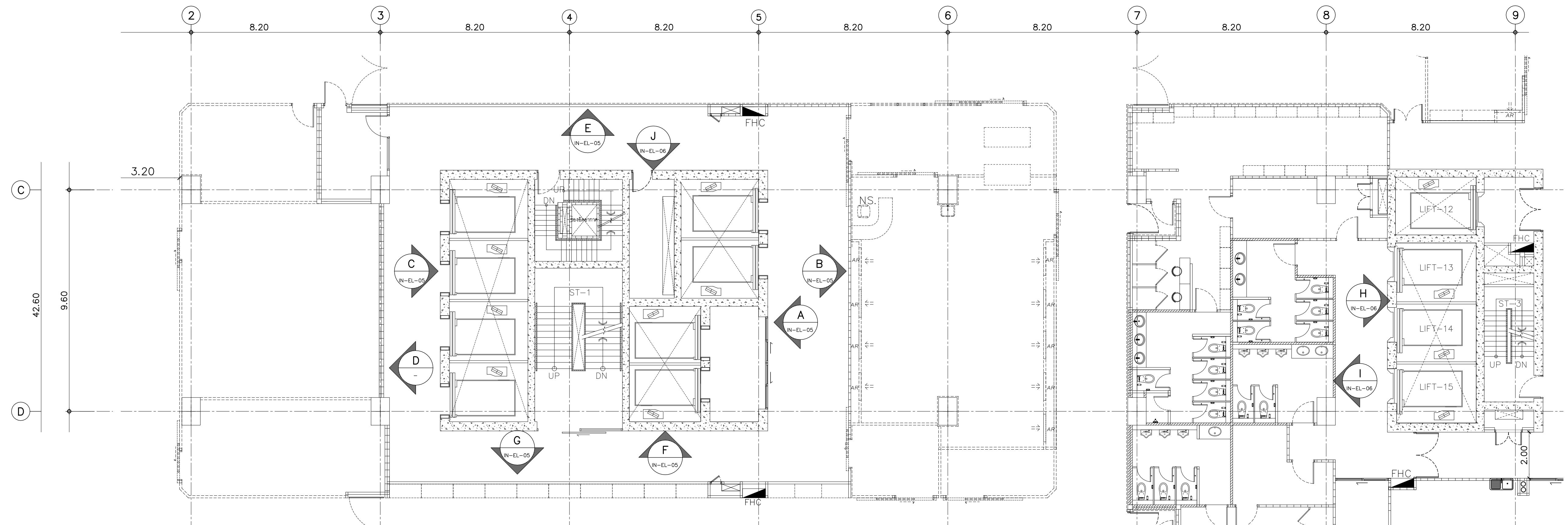
แผนผังเฟอร์นิเจอร์ชั้นที่ 4 มาตราส่วน 1:100
