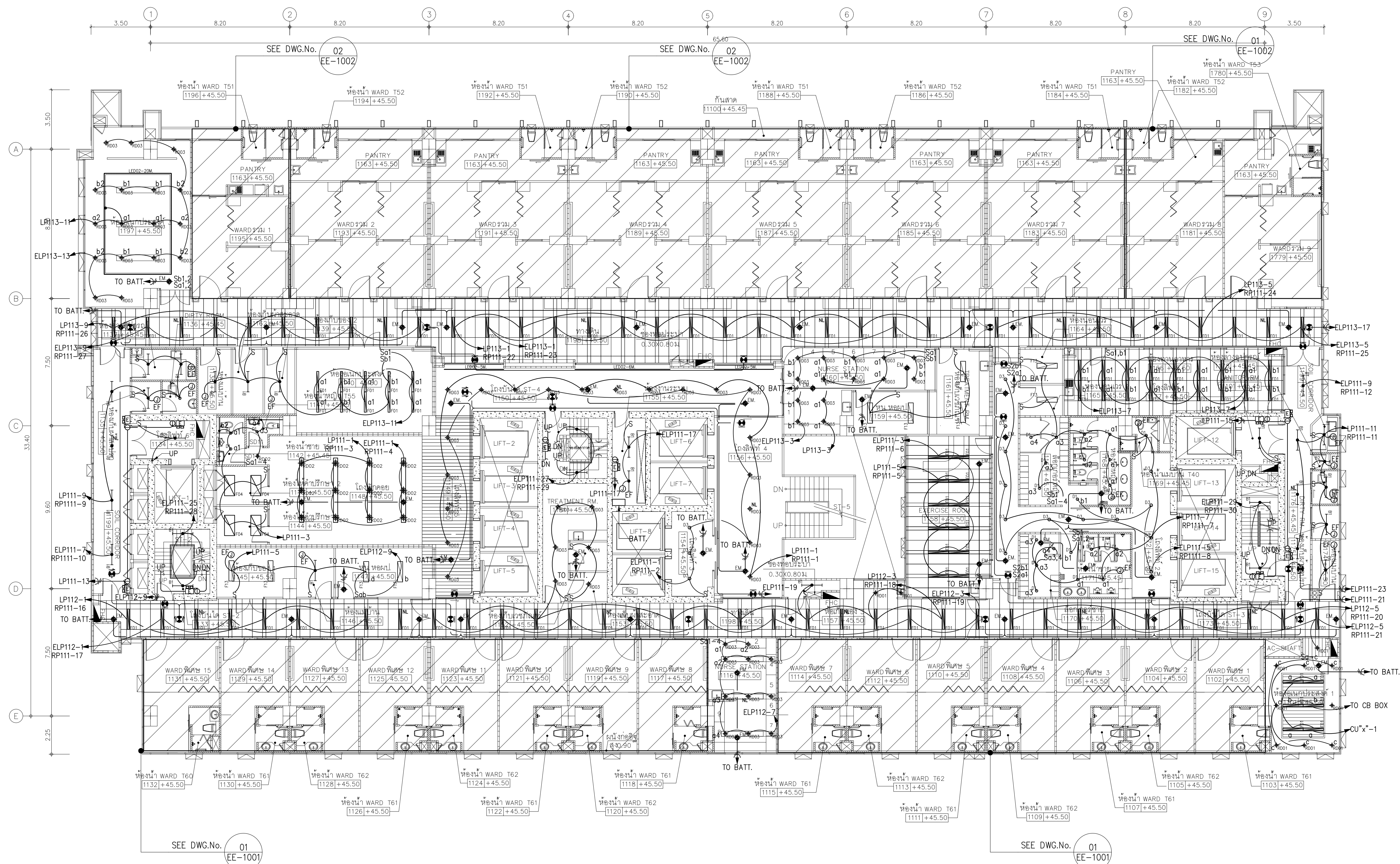
01 แปลนระบบไฟฟ้าแสงสว่างแสงสว่างฉุกเฉินและป้ายไฟทางออกฉุกเฉินชั้นที่ 11 A10 1:125 A30 1:250
