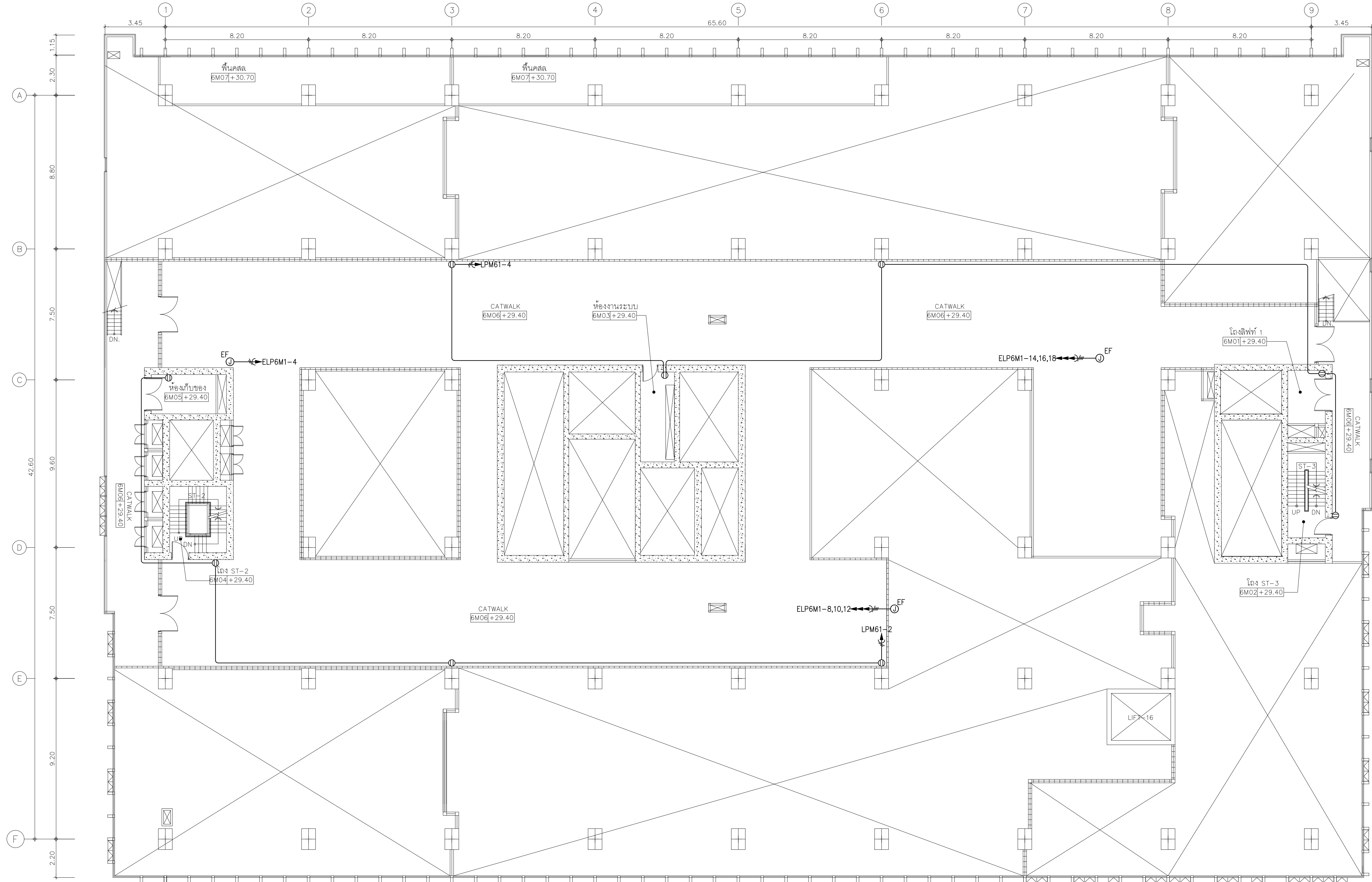
01 แผนระบบเตารับไฟฟ้าชั้นลอย 6M A1@ 1:125 A3@ 1:150 0 2 5 BAR SCALE
