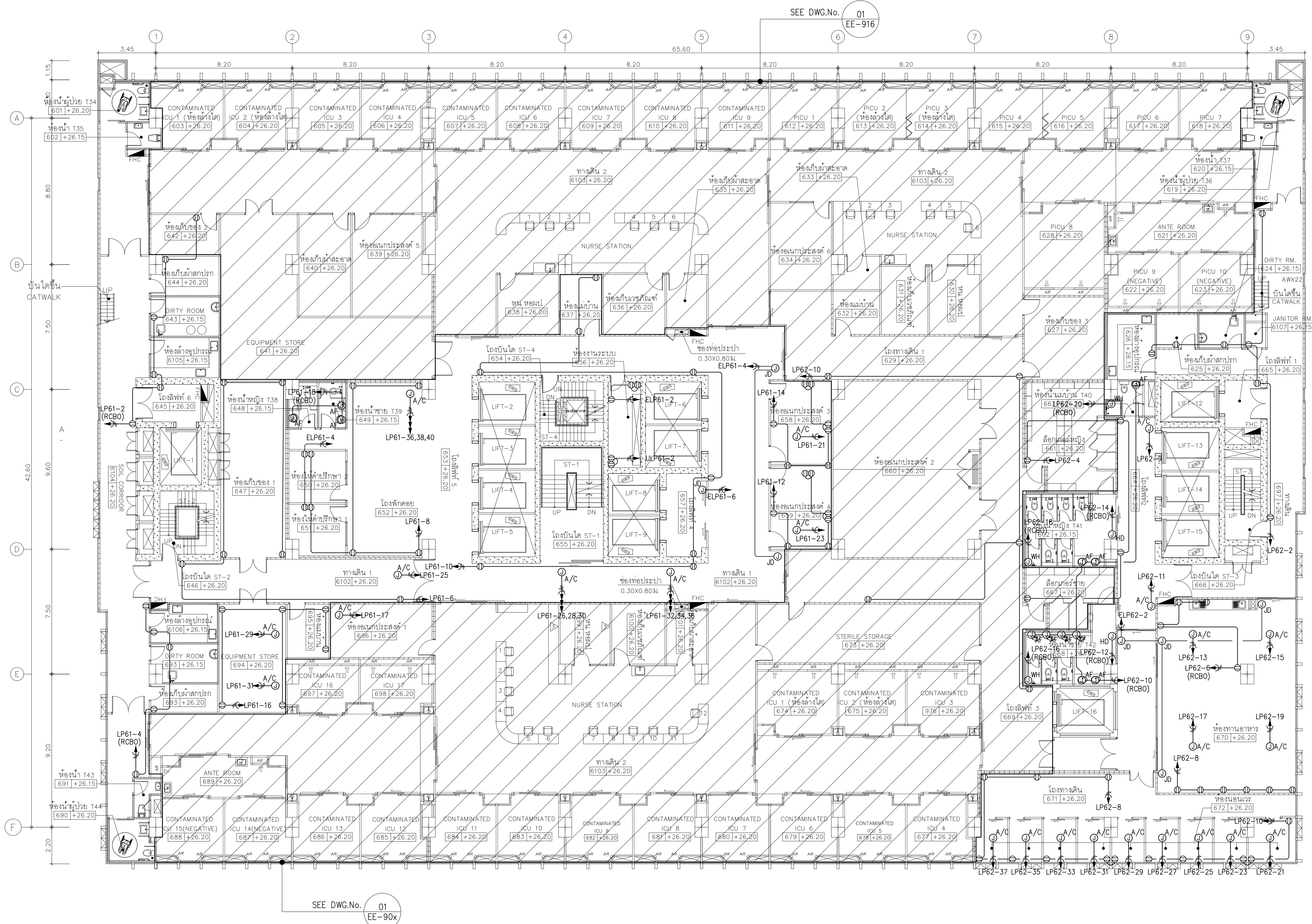
01 แปลนระบบเดินไฟฟ้าชั้นที่ 6 A10 1:125 A30 1:150 0 2 5 BAR SCALE
