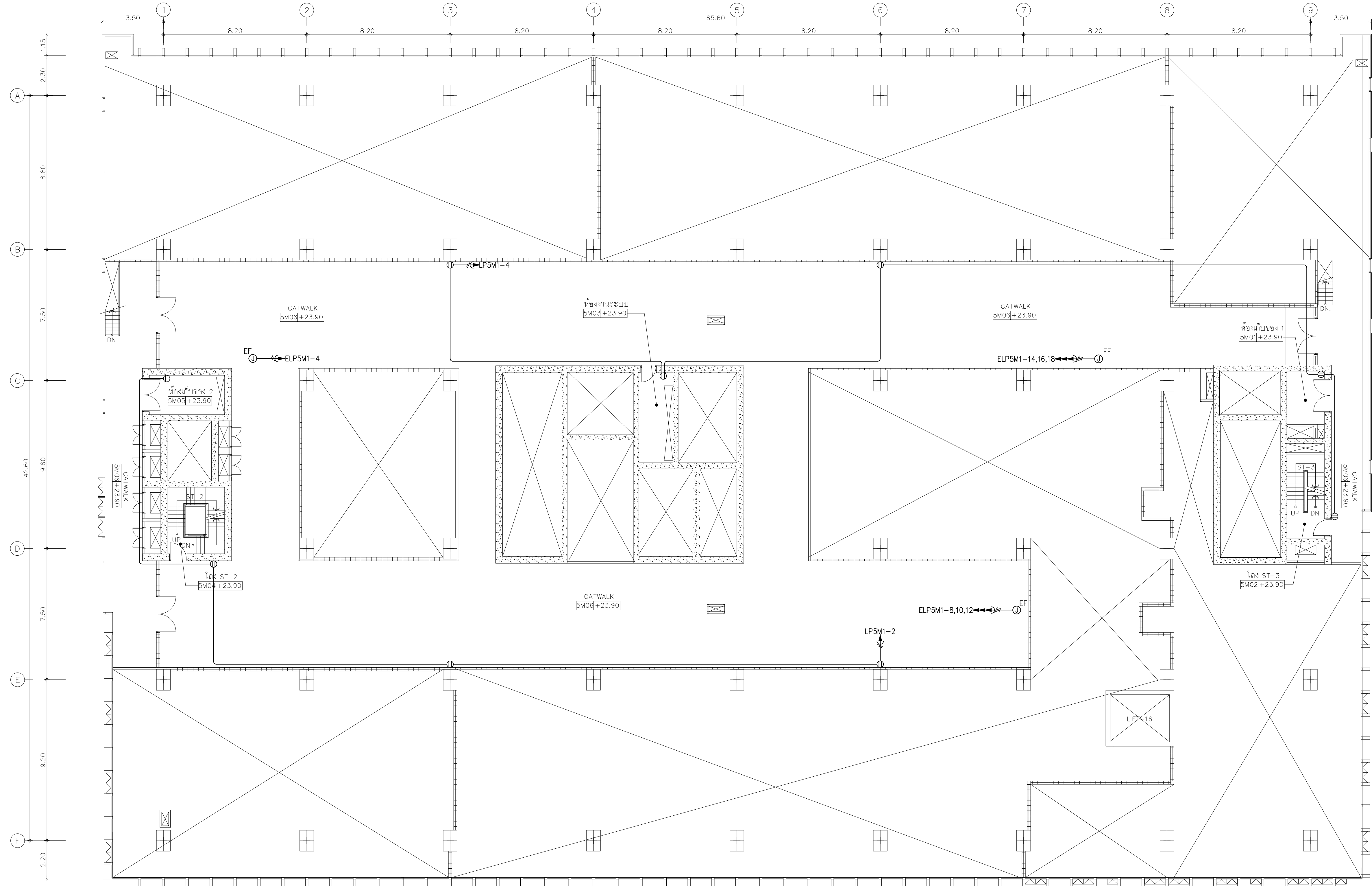
01 แผนระบบเดินไฟฟ้าชั้นลอย 5M A1@ 1:125 A3@ 1:150 0 2 5 BAR SCALE
