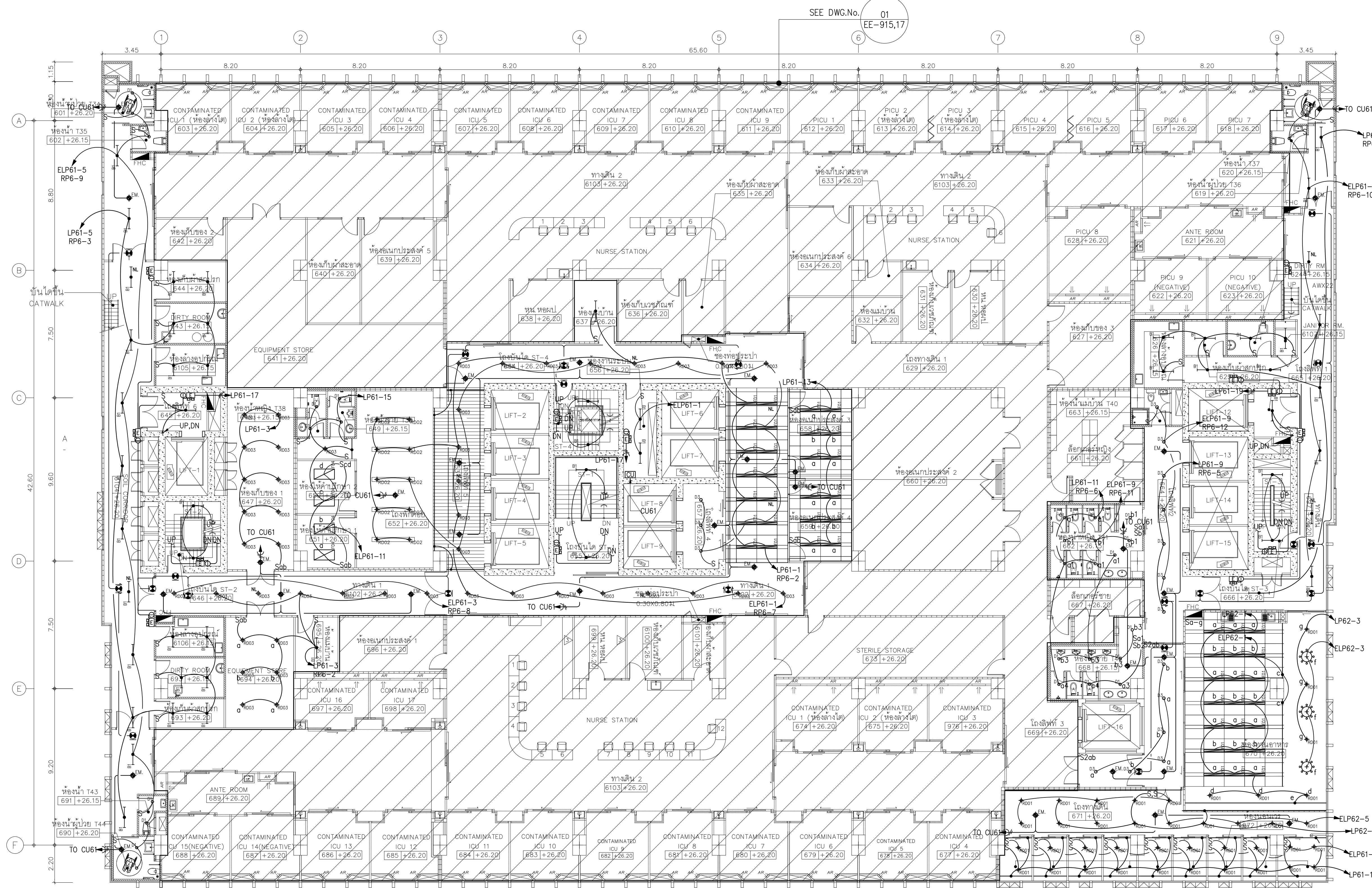
01 แปลนระบบไฟฟ้าแสงสว่าง แสงสว่างฉุกเฉินและป้ายไฟทางออกฉุกเฉินชั้นที่ 6 A10 1:125 A30 1:250 0 2 5 BAR SCALE
