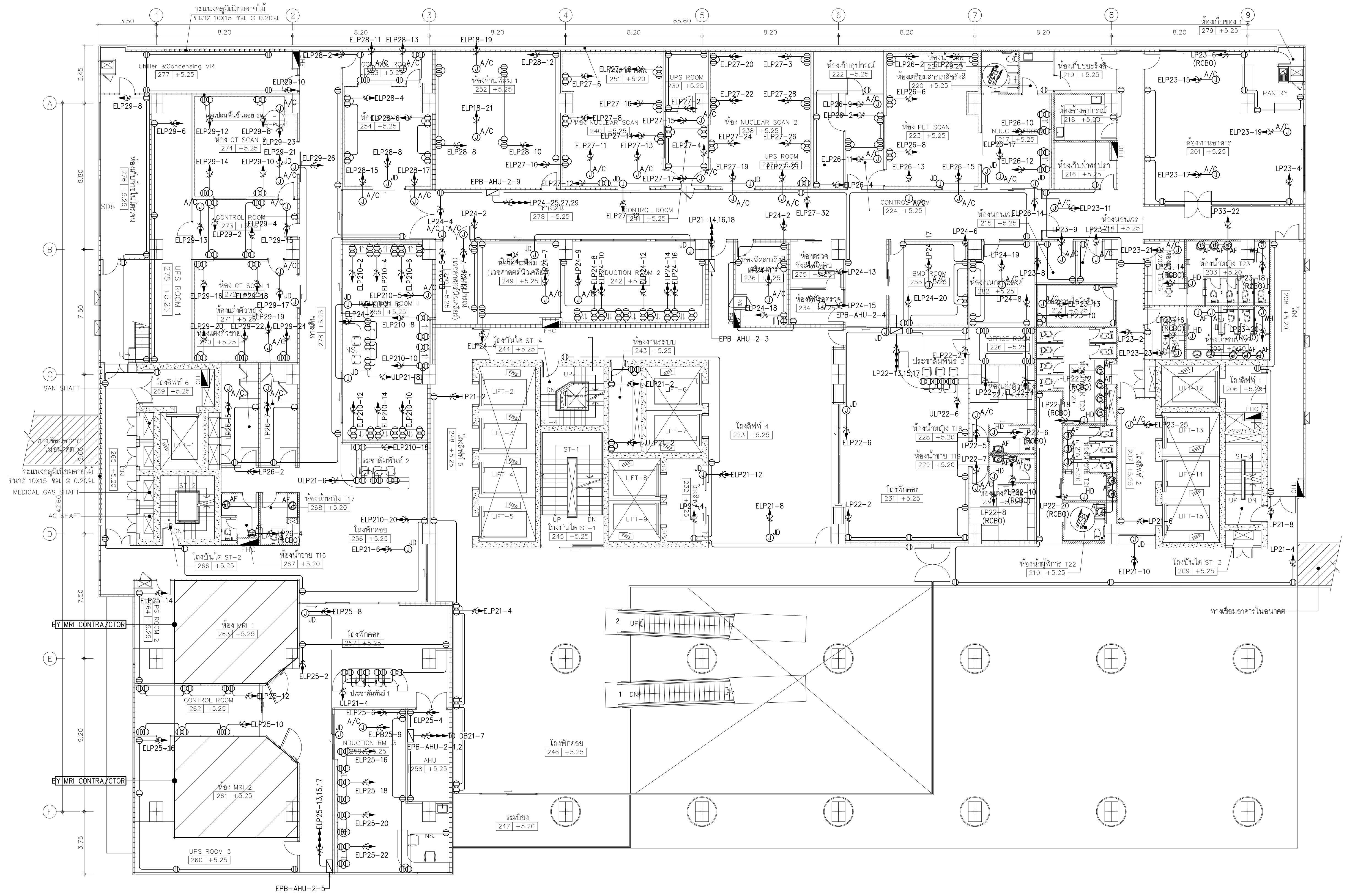
01 แผนระบบไฟฟ้าชั้นที่ 2 A10 1:125 A30 1:150 0 2 5 BAR SCALE
