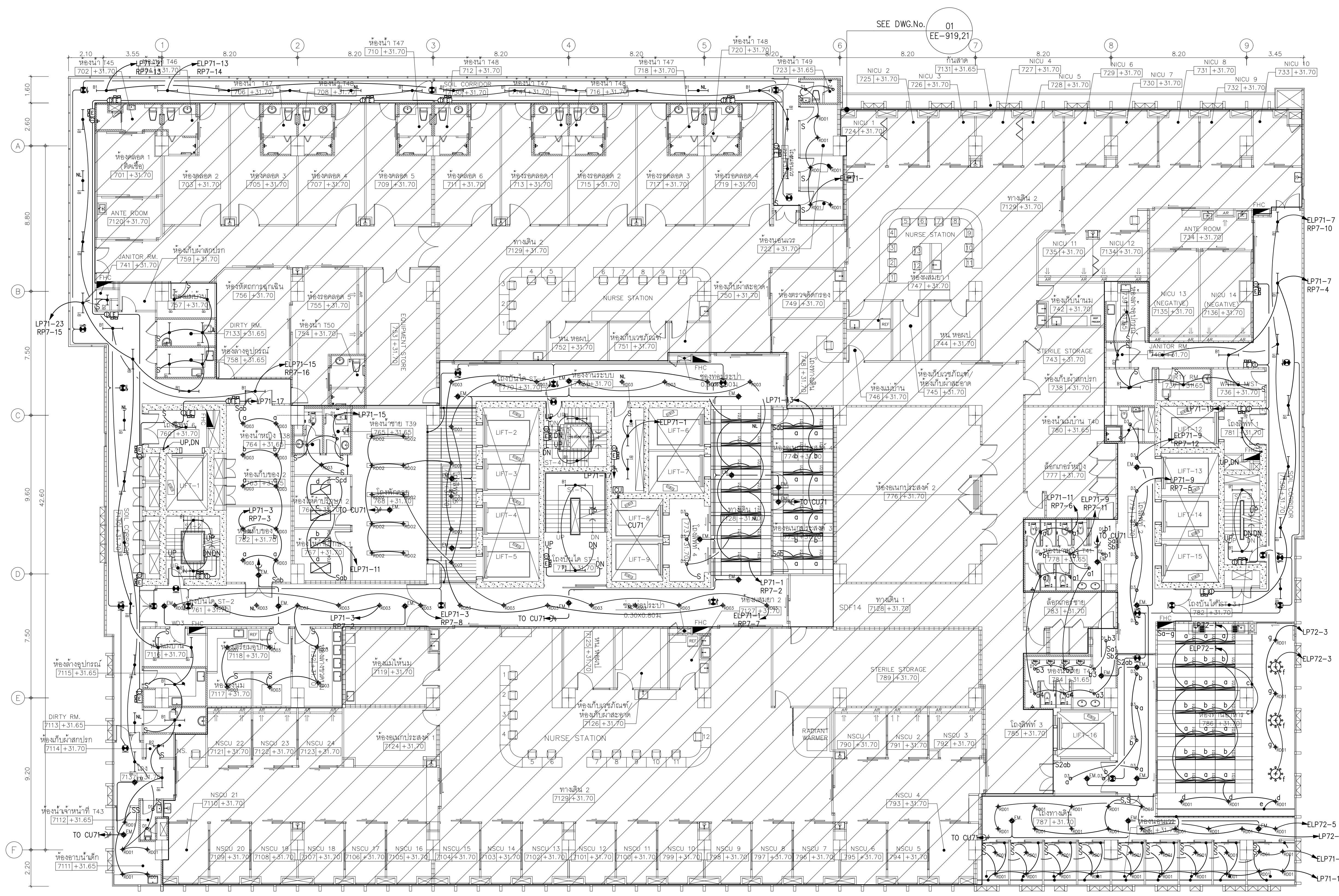
01 แปลนระบบไฟฟ้าแสงสว่าง แสงสว่างฉุกเฉินและป้ายไฟทางออกฉุกเฉินชั้นที่ 7 A10 1:125 A30 1:250 0 2 5 BAR SCALE
