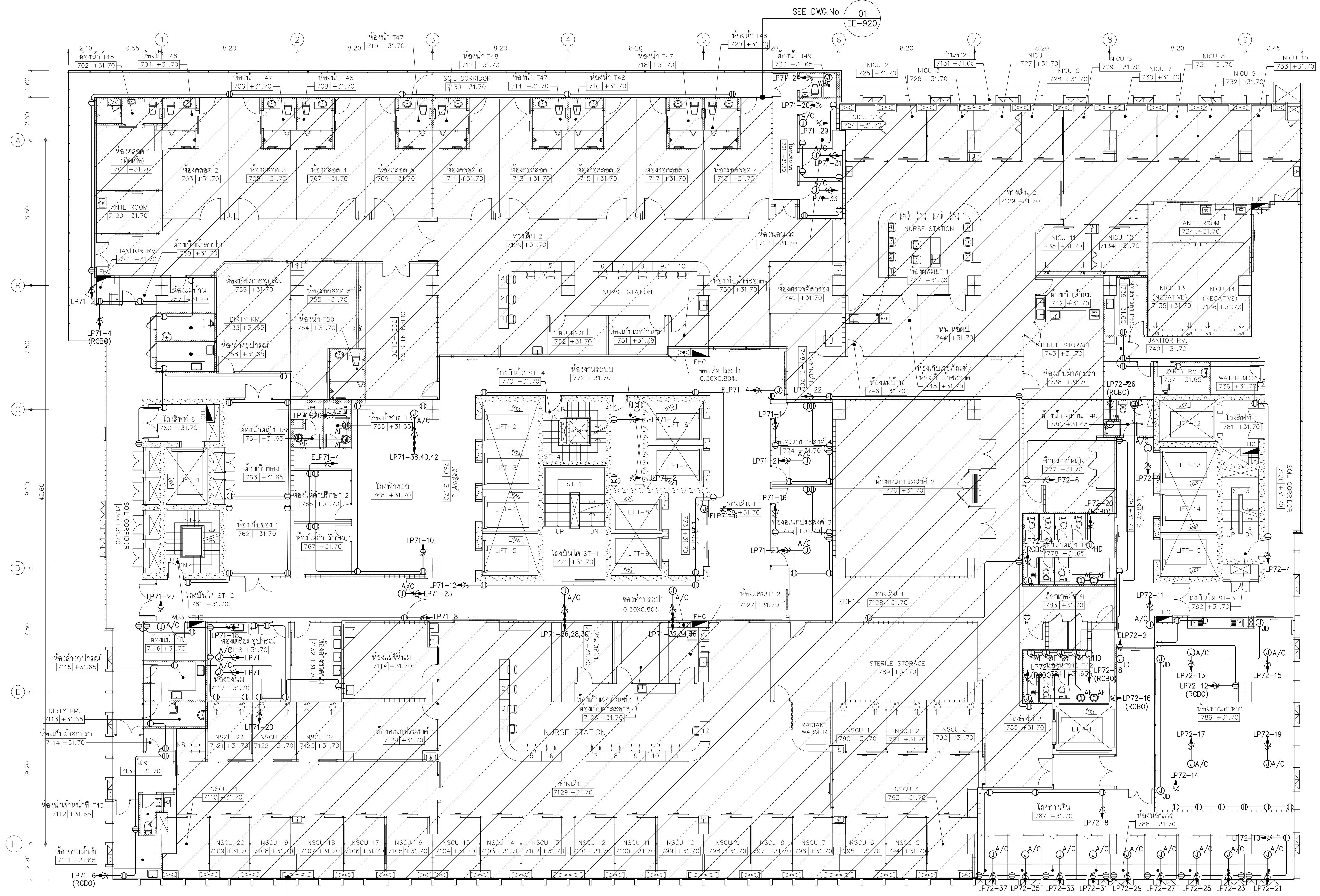
01 แผนระบบเดินไฟฟ้าชั้นที่ 7 A10 1:125 A30 1:150 0 2 5 BAR SCALE
