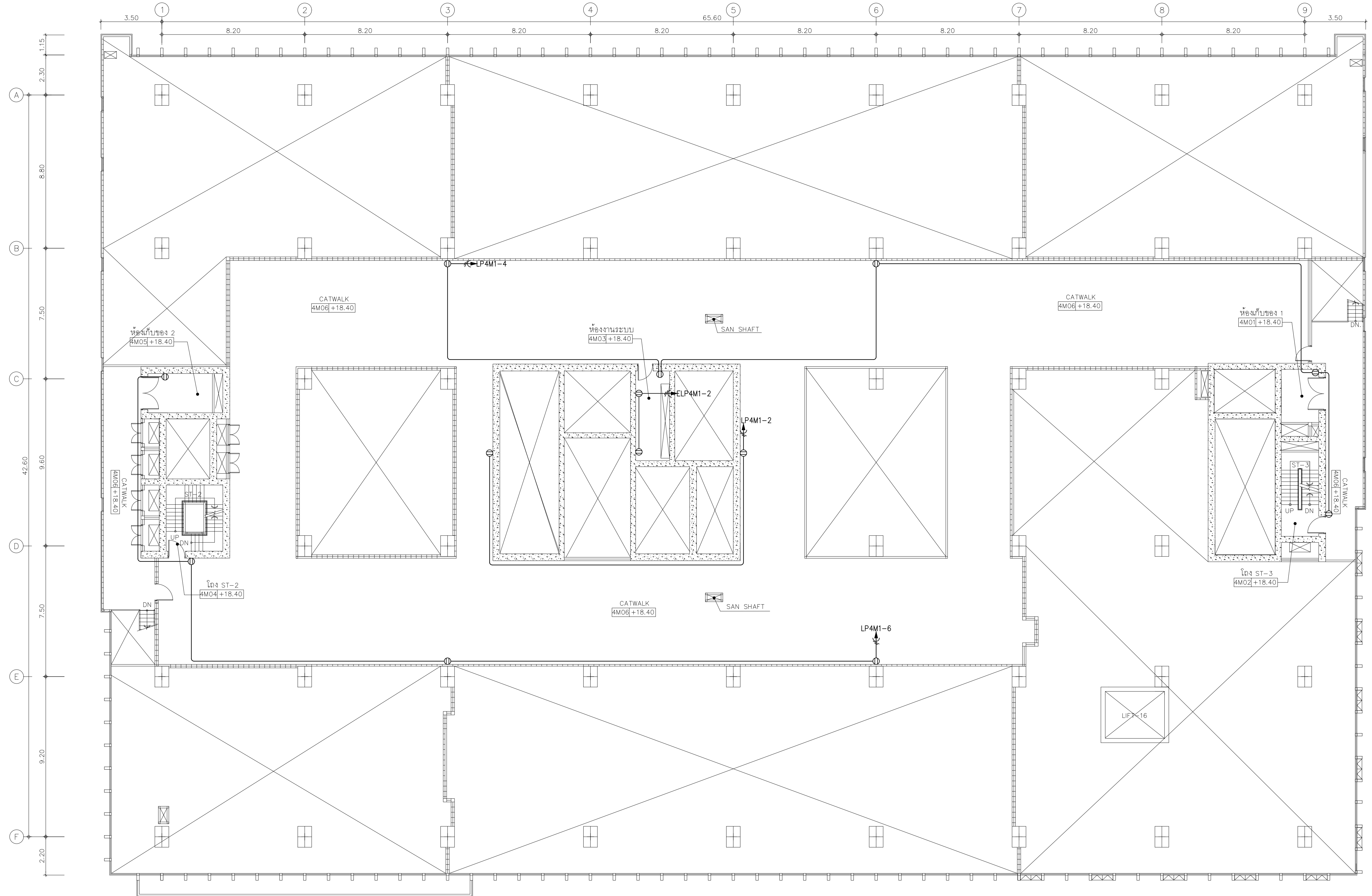
01 แปลนระบบเดินไฟฟ้าชั้นลอย 4M A1@ 1:125 A3@ 1:150 0 2 5 BAR SCALE
