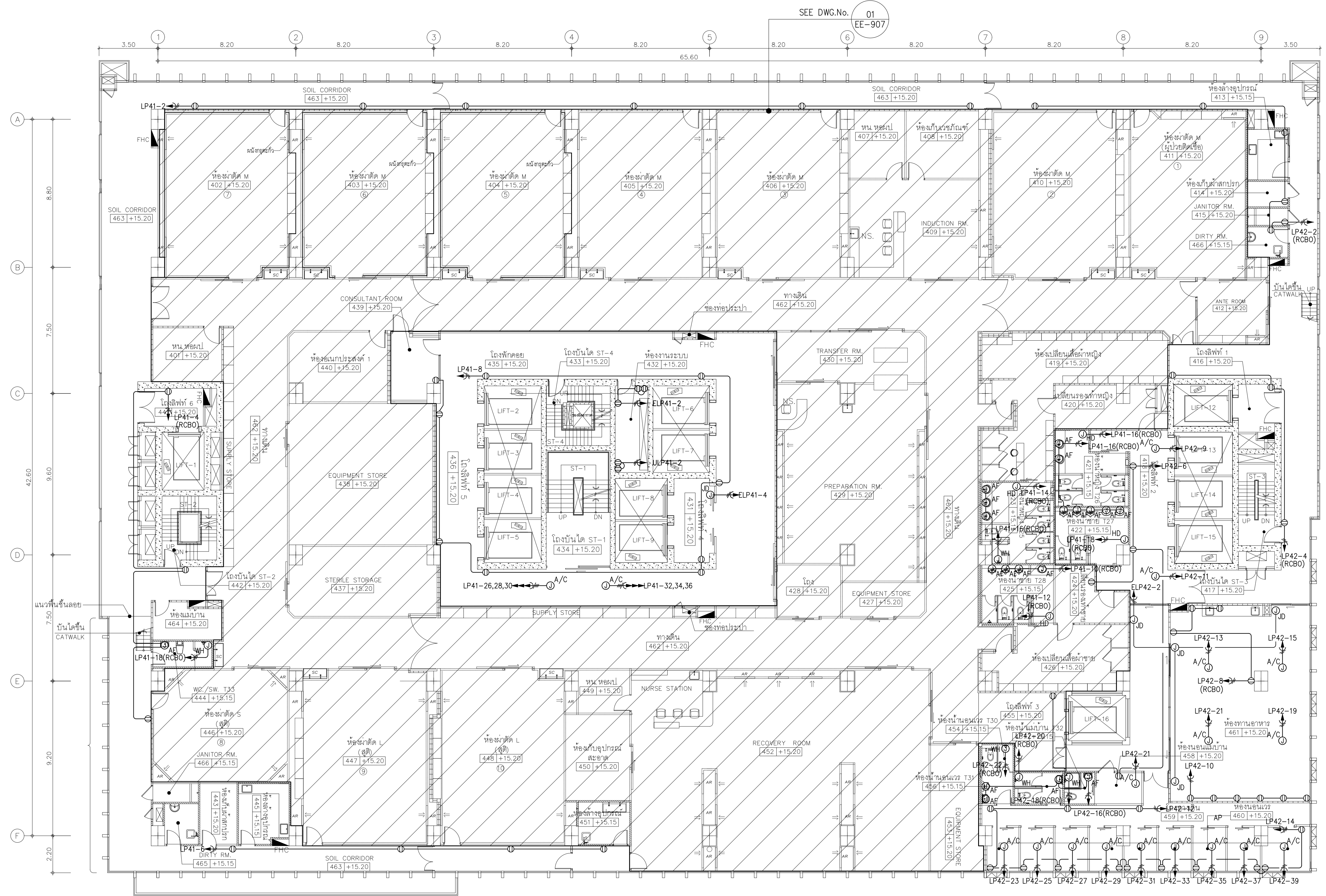
01 แปลนระบบเดินไฟฟ้าชั้นที่ 4 A10 1:125 A30 1:150 0 2 5 BAR SCALE
